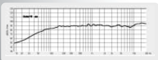
Réponse en fréquence / Frequency response
