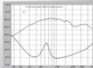
Réponse en fréquence & impédance en mode passif Frequency response & impedance in passive mode
